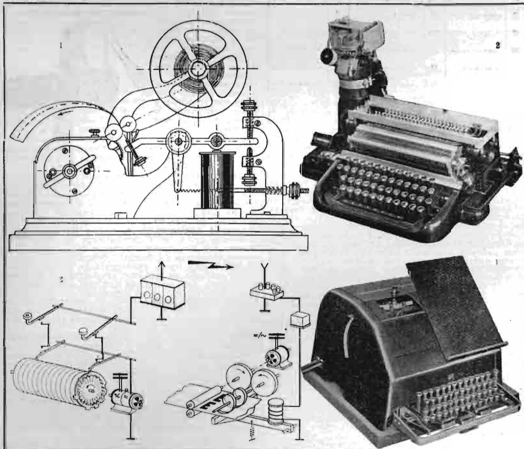
1. Морзев апарат. — 2. Хелов апарат. — 3. Шема предајног и пријемног Хеловог а. — 4. Старт-стоп телегр. апарат.
