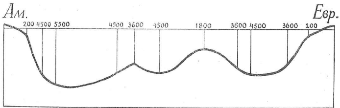
Сл. 11. — Профил дна Атлантског Океана,
