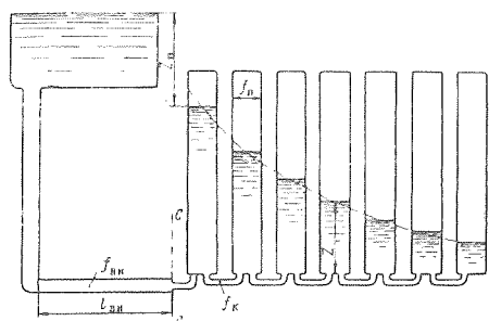
Хидроинтегратор из 1937.
