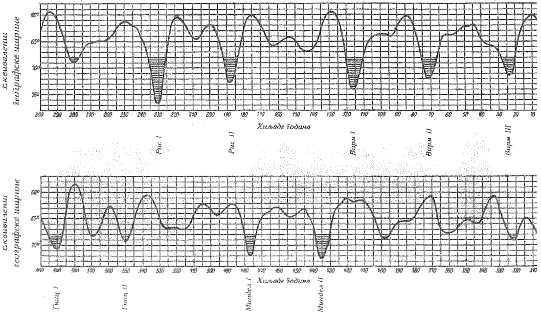
Слика 10. Миланковићева крива осунчавања. На апсциси је време од данашњег тренутка обележеног са 0 до 600.000 година уназад, а на ординати је еквивалентна ширина која показује којој данашњој географској ширини одговара осунчавање на ширини 65^\circ у неком тренутку прошлости.
