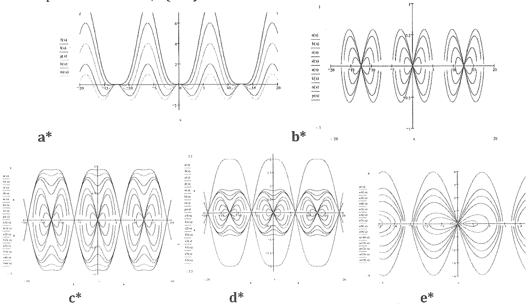
Слика10. Параметарска трансформација фазних трајекторија и хомоклиничких орбита ( b* ) – ( e* ) релативног кретања тешке материјалне тачке по ротирајућој, кружној глаткој линији, константном угаоном брзином око вертикалне осе (за модел на слици 9.b*, за \epsilon=0 ) при промени угаоне брзине ротације. ( a* ) график аналогу потенцијалне енергије система.
