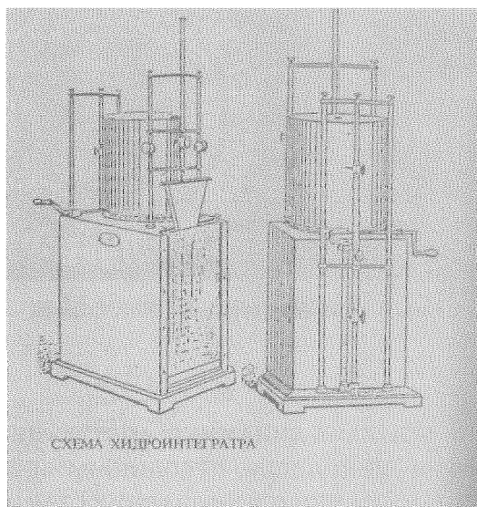
Слика 7. Сlike модела хидроинтегратора Михаила Петровића Аласа [66].
