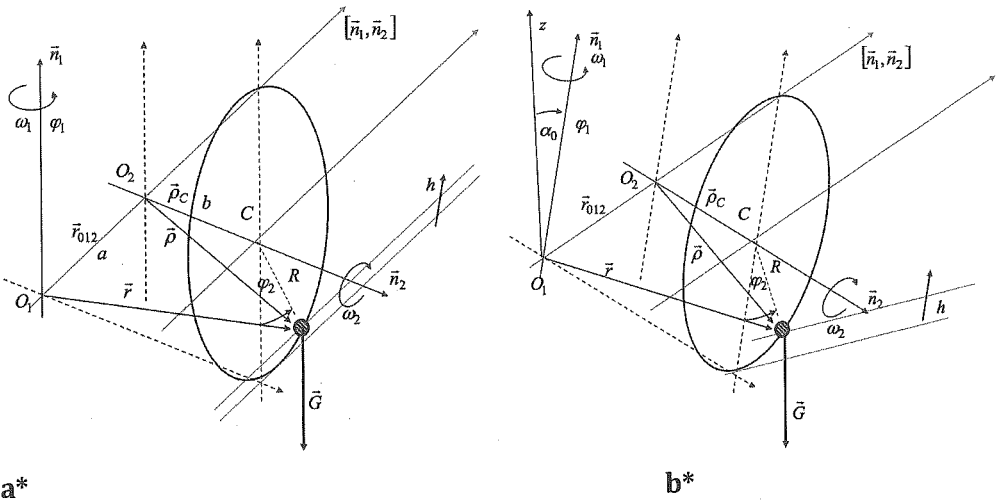
Слика 11. Кретање тешке материјалне тачке спрегнутим ротацијама око ортогоналних мимоилазних оса, од којих је фиксирана оса вертикална (а*), односно коса у односу на вертикалу (б*).
