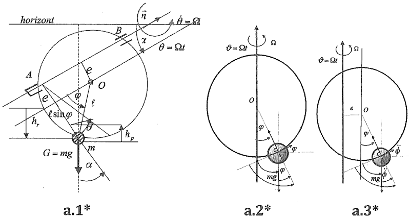
Слика 9. a* Модели тешке материјалне тачке која се креће по ротирајућем кругу, константном угаоном брзином, око ексцентричне осе косо постављене у односу на хоризонт (a*1), односно вертикалне центричне (a*2) или вертикалне ексцентричне осе (a*3).
