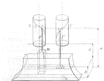
Принцип хидроинтегратора из 1897.
