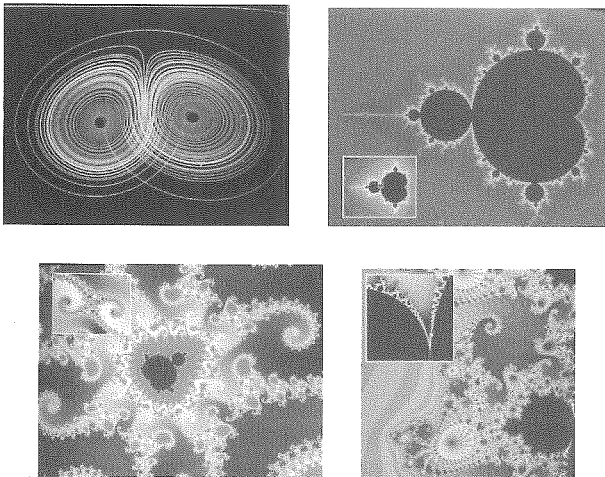
Слика 3. Лоренцов атрактор и леви фрактални скупови [3]
