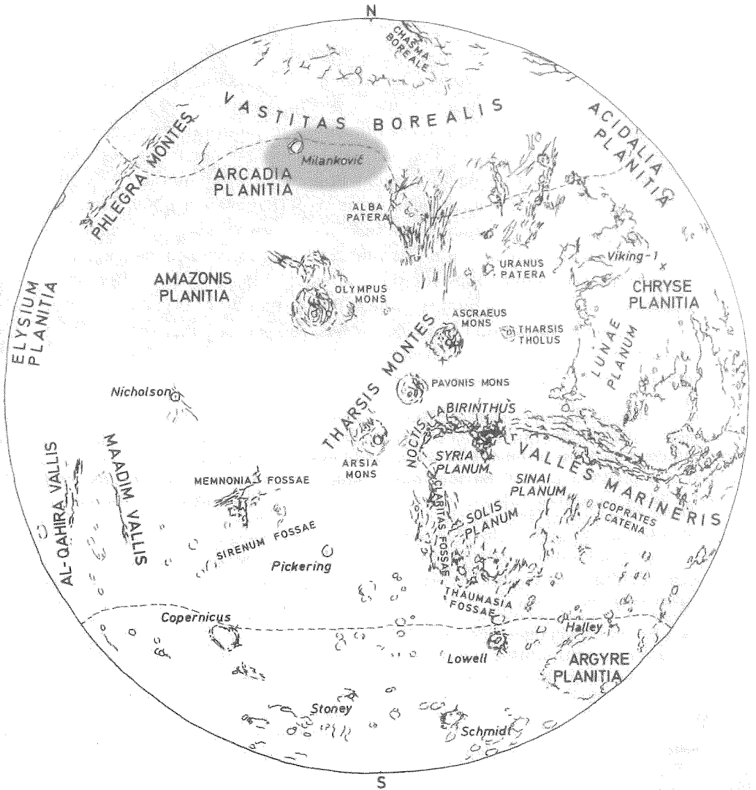
Слика 13. Кратер Миланковић на Марсу (Вујновић, 1989)
